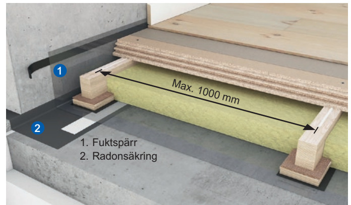
Figur 1 Undergolv på betongdäck ska alltid utföras med fuktspärr och radonspärr på betongytan.
